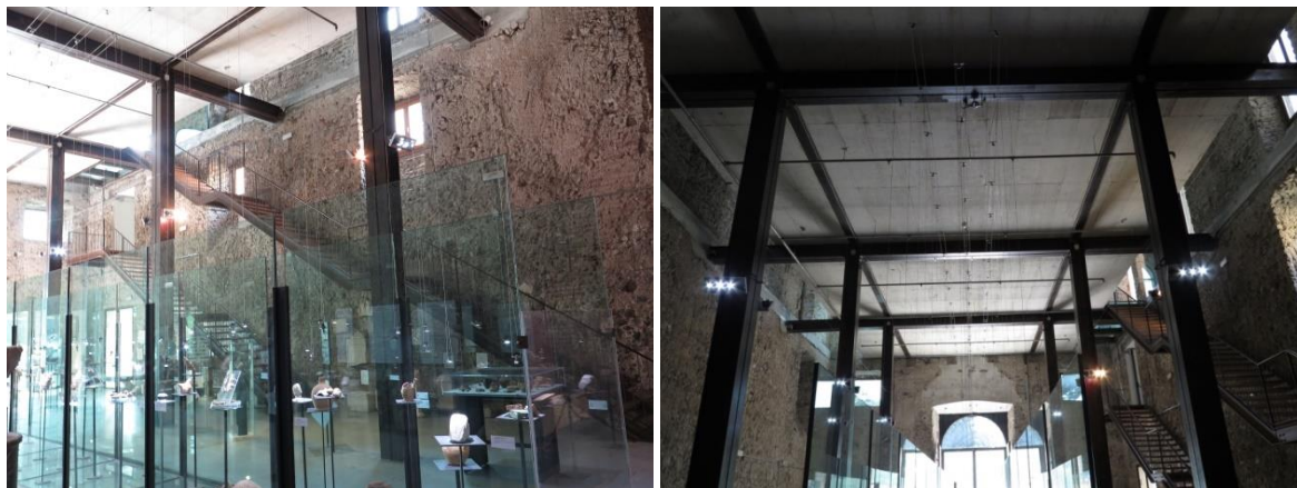
Figura 6 – Antiquarium Tuscolano na Scuderie Aldobrandini, Frascati. Massimiliano Fuksas. Fotos: Betânia Brendle, 2015.
